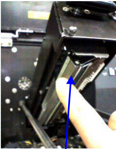
剥離版が降りた状態（金箔リボン用）
